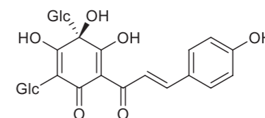
safflorin A
