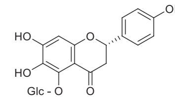
neocarthamin
