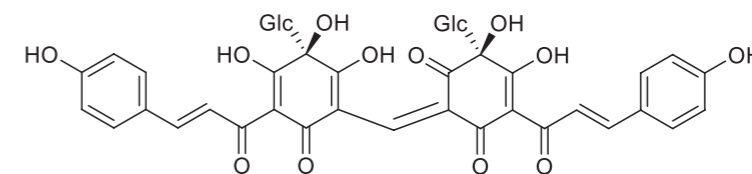
carthamin
