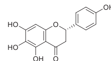
carthaminidin
